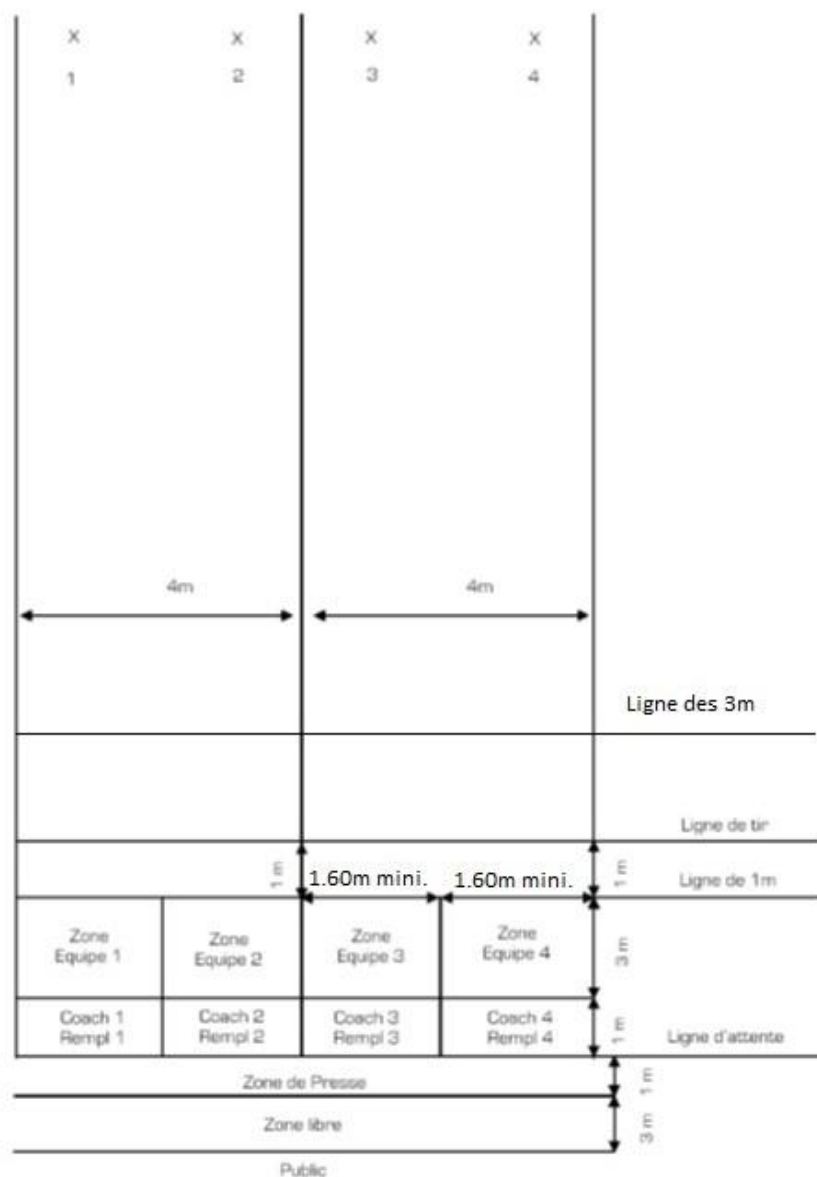
AMENAGEMENT DE LA LIGNE DE TIR POUR LE TIR PAR EQUIPES
